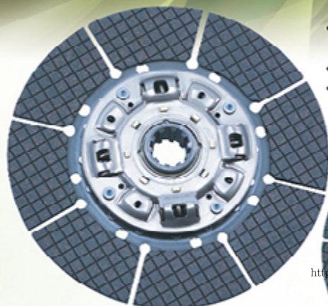
油式離合器 Wet-type Clutches
