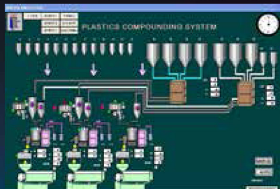
全自動原料計量輸送膠粒製造系統 Automatic Ingredient handling compounding system
