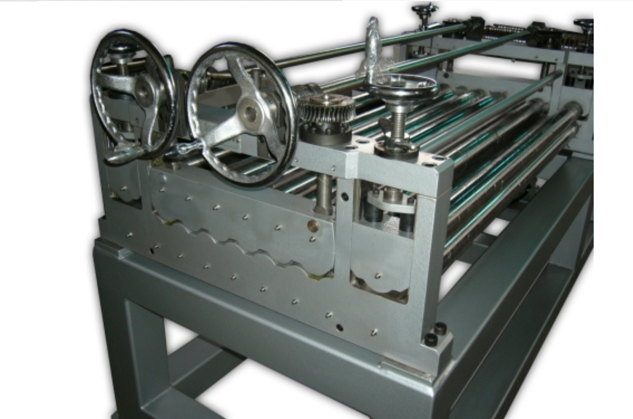
LEVELLER
