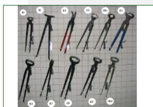
Forging Farriertools
