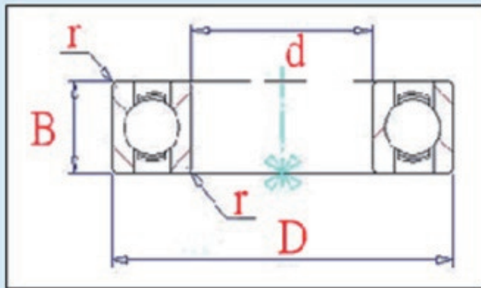
Deep Groove Ball
