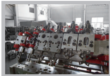
COMBO TRANSFER 複合式傳送機構
