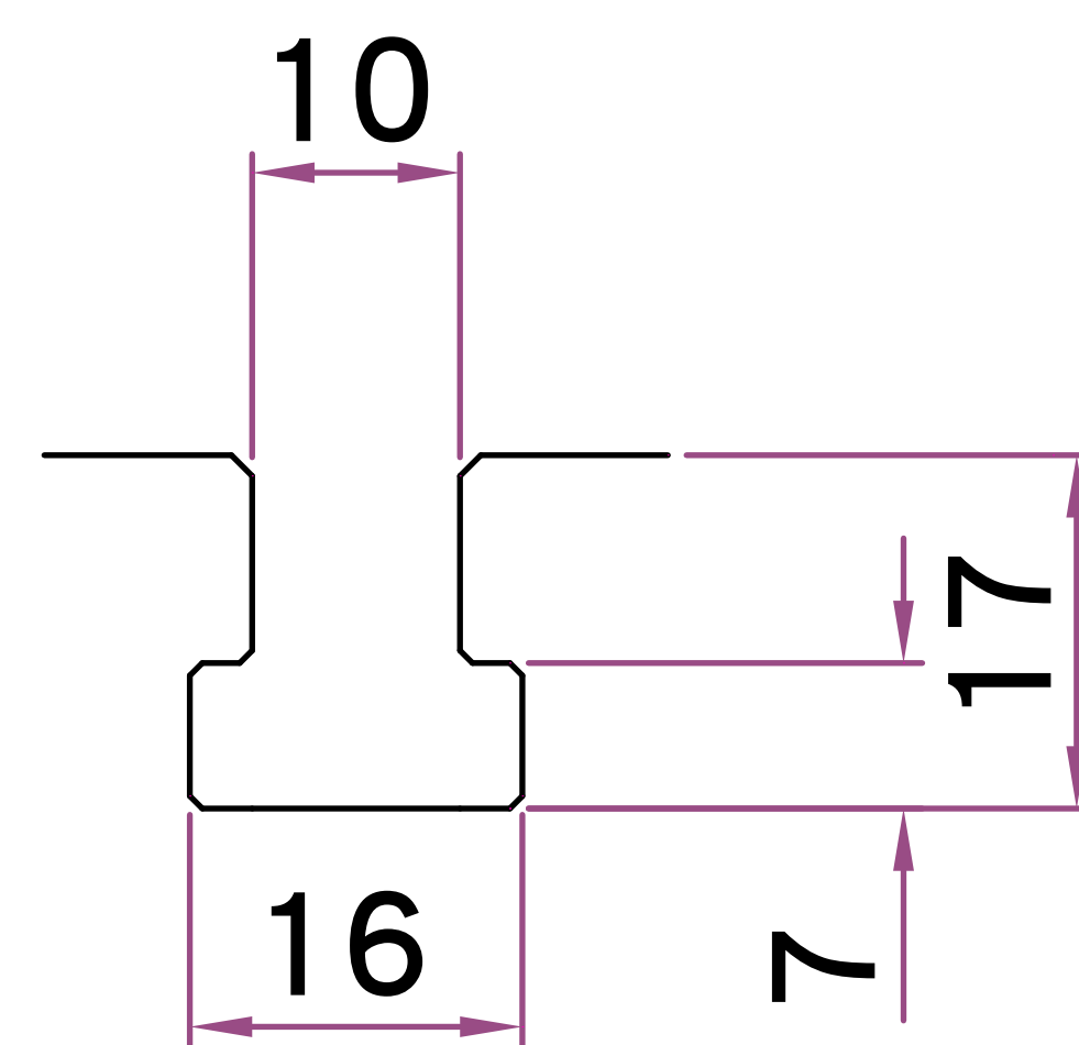
T 型槽尺寸
